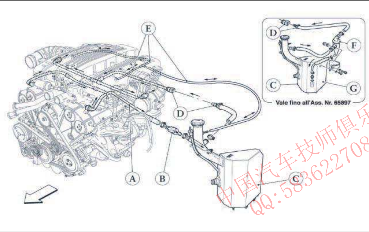
机油蒸气再循环系统图
